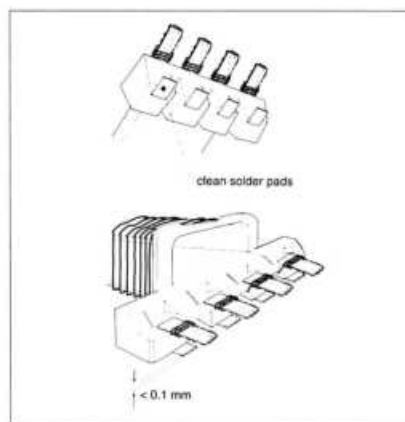
Afb. 2. 'U-pin'-aansluitingen.
